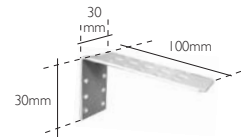
Soporte de instalación a techo
